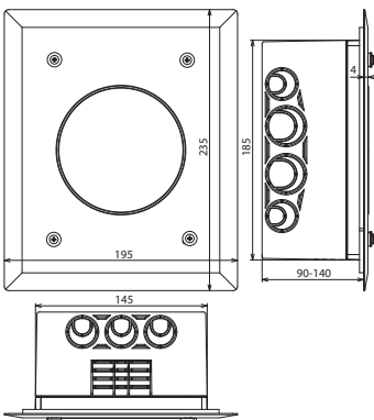
Maßbild TSK WDVS 180X140X88 K V2A
