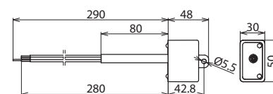
Maßbild DCOR L 2P 275 SO IP
