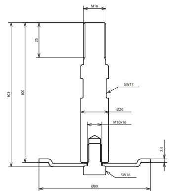
Maßbild FS TE 20 100 M16 FP80 STTZN
