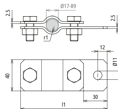
Maßbild ERS 27 AB11 V2A
