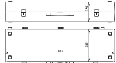
Maßbild FRS ZK MS
