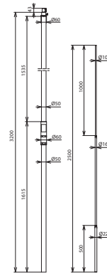
Maßbild SR D50 3200 FS22 2500 IP HVI GFK
