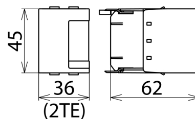
Maßbild DSE MOD PE 60
