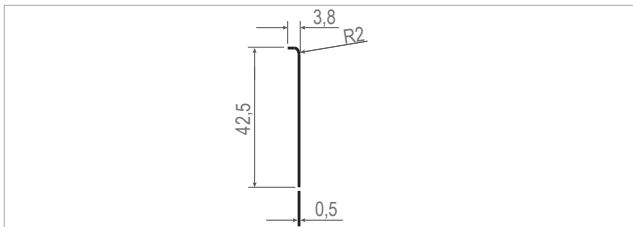
Metallhaken
