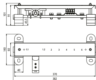
Maßbild PAS EX 7AP SET
