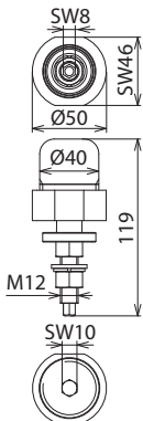
Maßbild MA SDS M12
