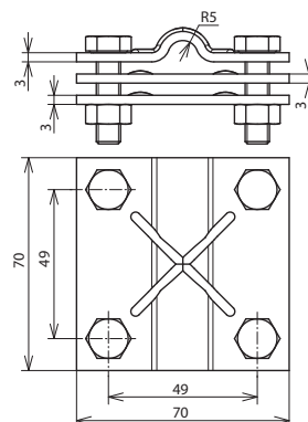
Maßbild KS 8.10 FL40 STTZN
