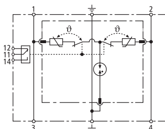
Prinzipschaltbild DR M 2P 75 FM
