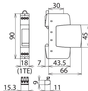
Maßbild DR M 2P 75 FM
