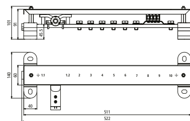
Maßbild PAS EX 11AP SET
