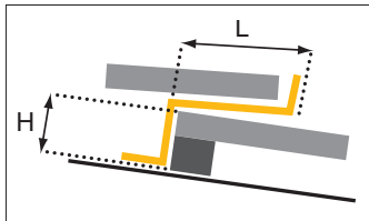
Skizze: Dachbefestigung Ziegel
